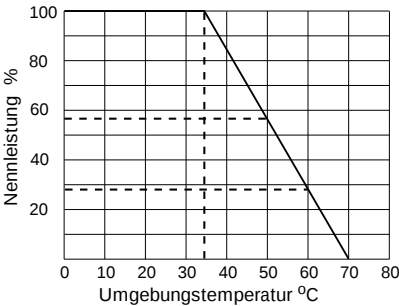
Anschlußleistung / Umgebungstemperatur-Diagramm
