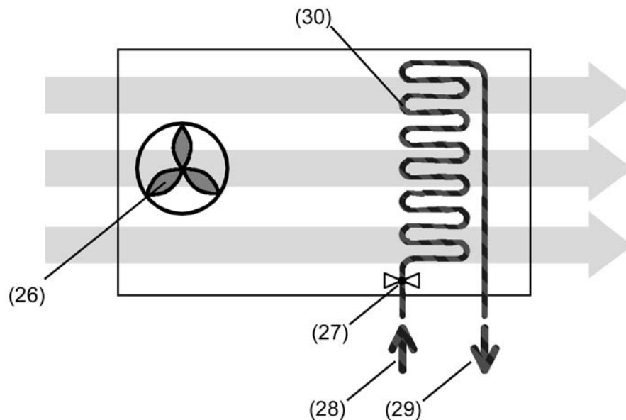
Bild 8: Das 2-Rohr-System
