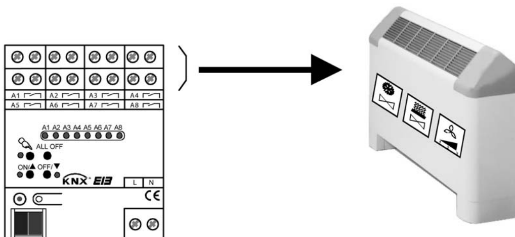
Bild 10: Der 1-Kanal-Betrieb
