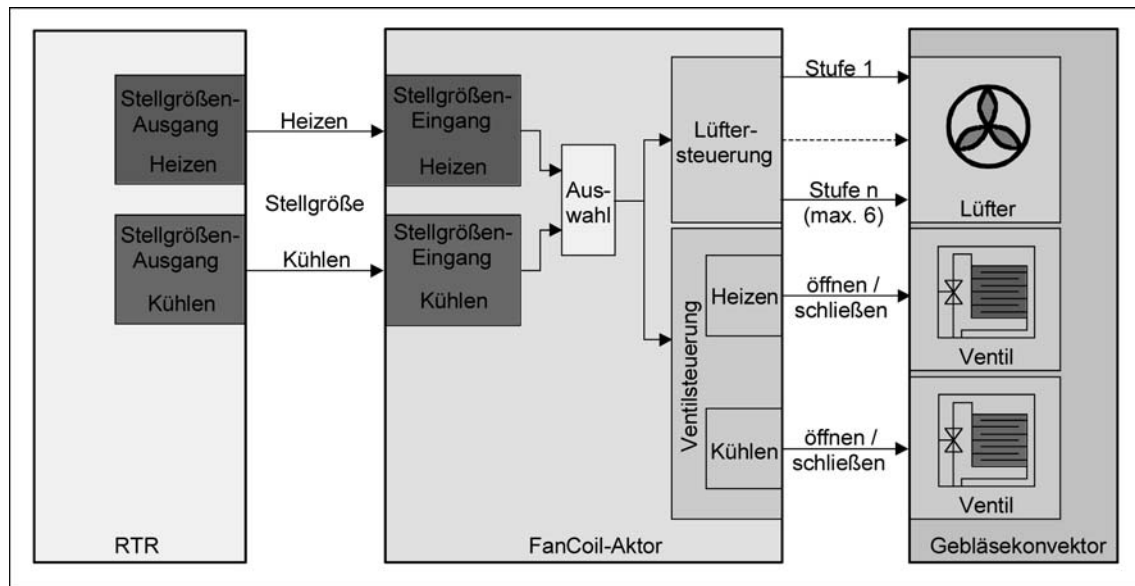
Bild 15: Funktionsschema "4-Rohr Heizen/Kühlen über Stellgrößenvorgabe"
