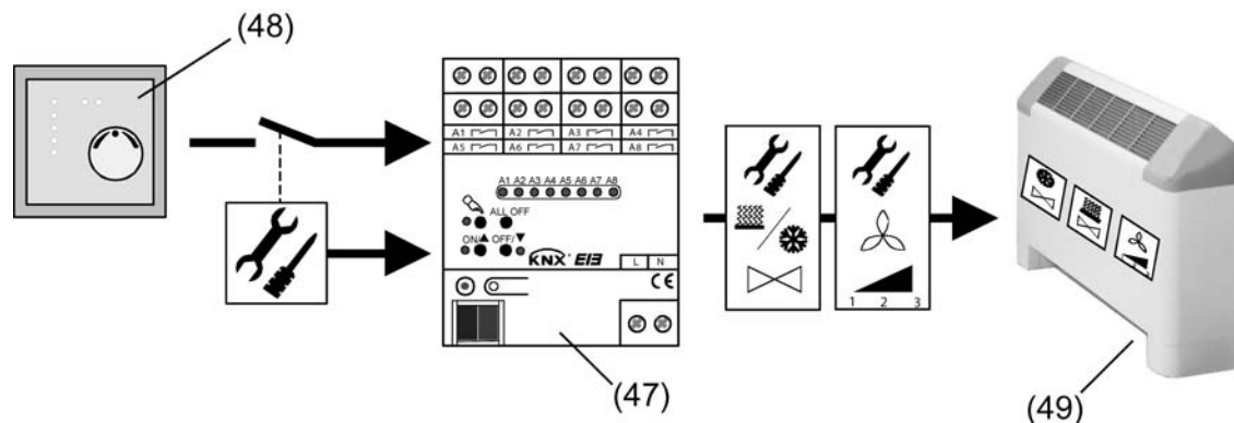
Bild 32: Prinzip der Sperrfunktion am Beispiel einer Wartungsverriegelung
