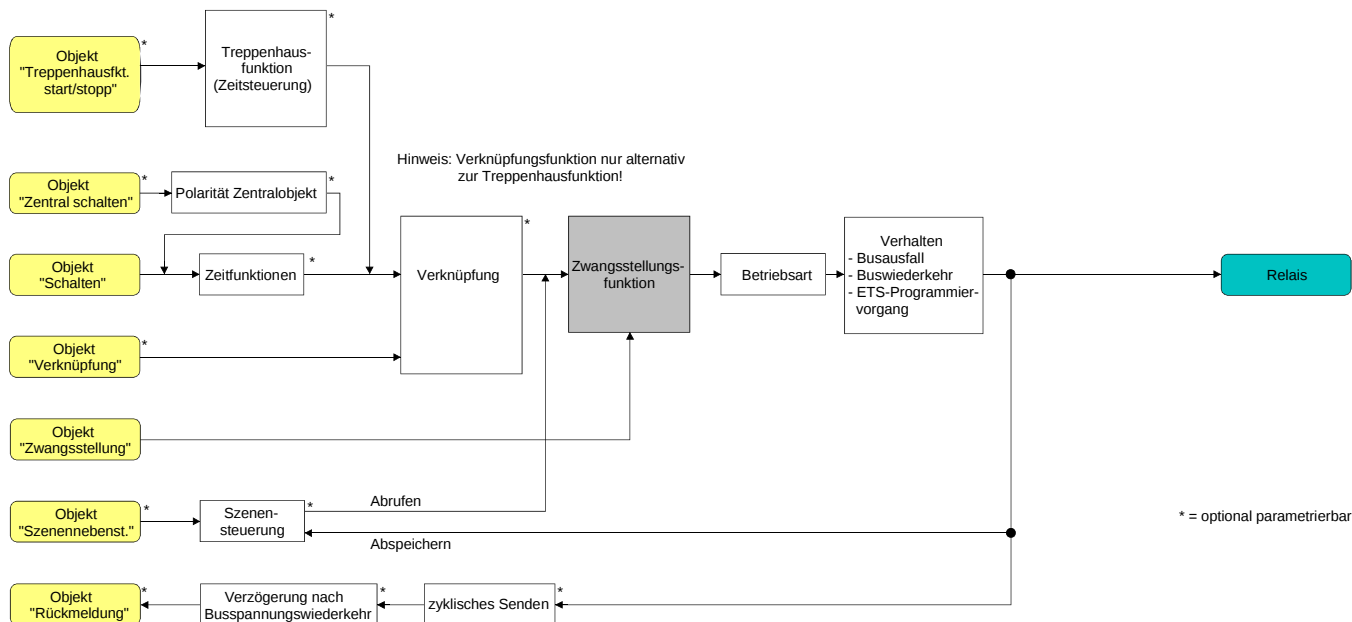
Bild 20: Funktionsschaltbild der Zwangsstellungsfunktion
