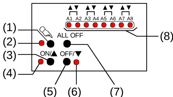
Bild 5: Bedien- und Anzeigeelemente der Handbedienung beim Schalt-/Jalousieaktor 4/8fach
