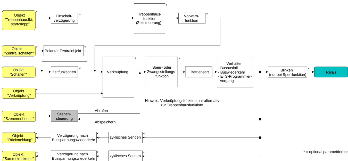
Bild 18: Funktionsschaltbild der Szenenfunktion
