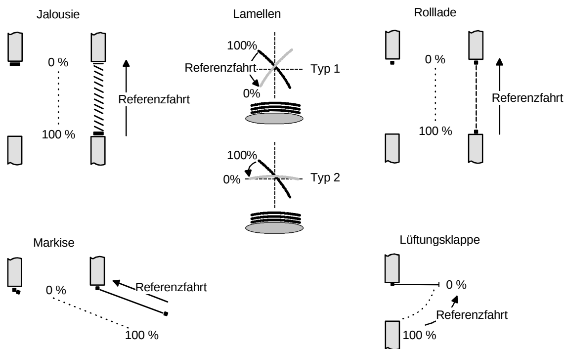
Bild 29: Referenzfahrt
