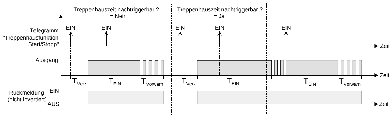
Bild 15: Einschaltverhalten der Treppenhausfunktion
