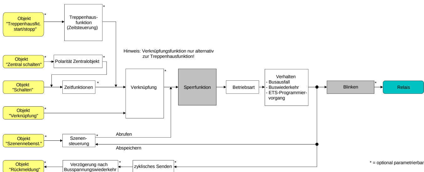
Bild 19: Funktionsschaltbild der Sperrfunktion
