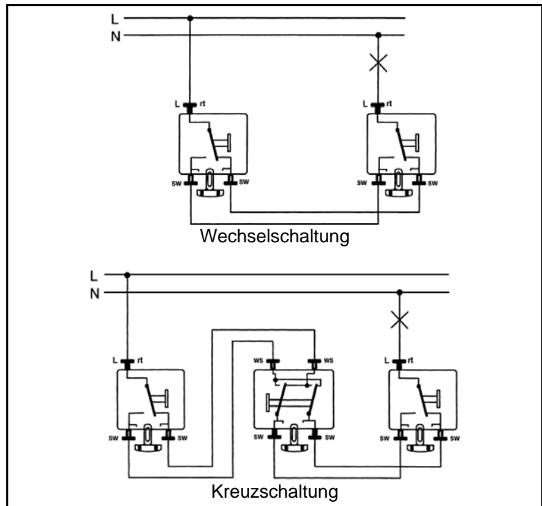
Anschlussbeispiel 506 U
