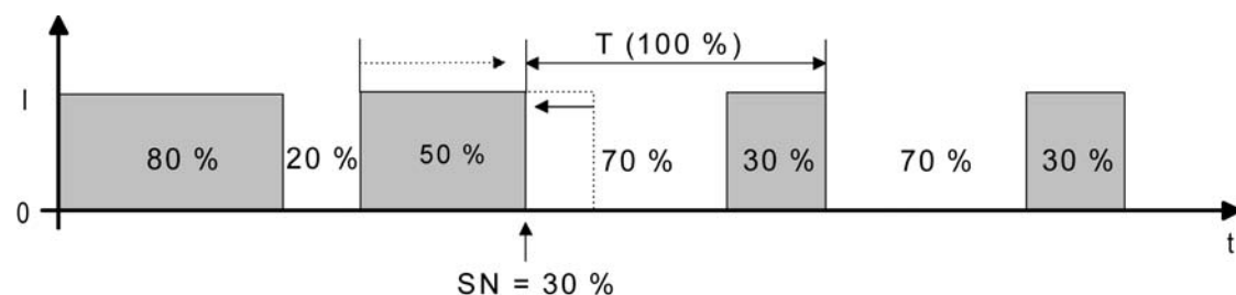
Bild 19: Stellgrößenänderung z. B. von 80 % auf 30 % während Öffnungsphase des Ventils (Öffnungsphase zu lang)
